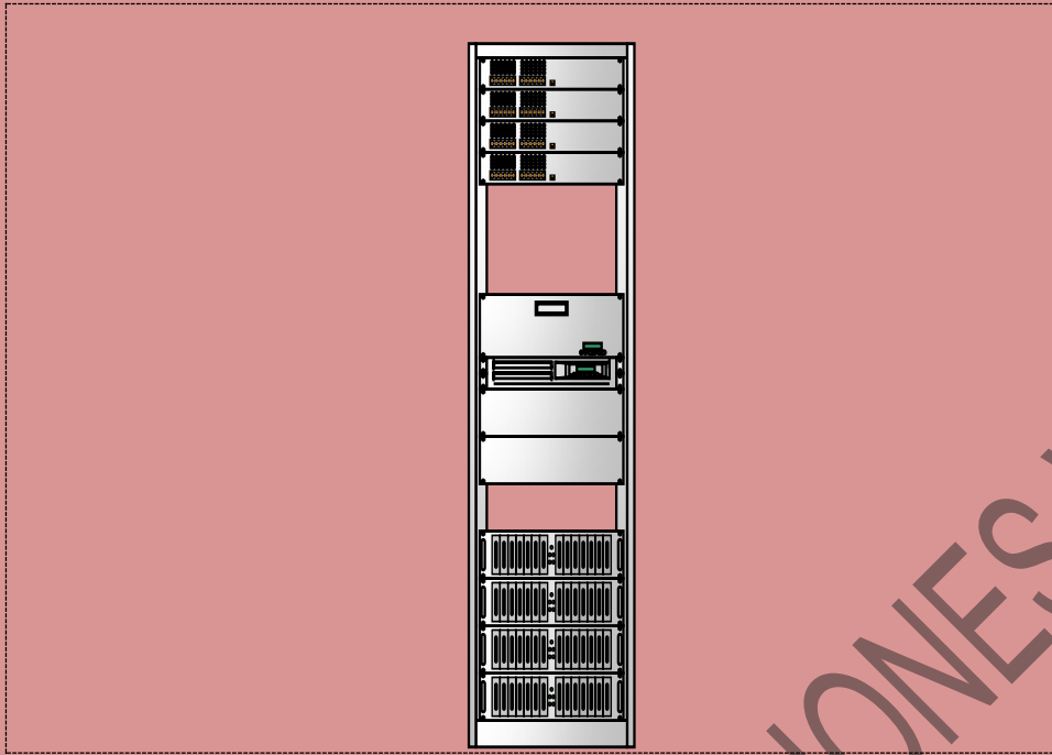
Imagen 1. Distribución Física SAN
