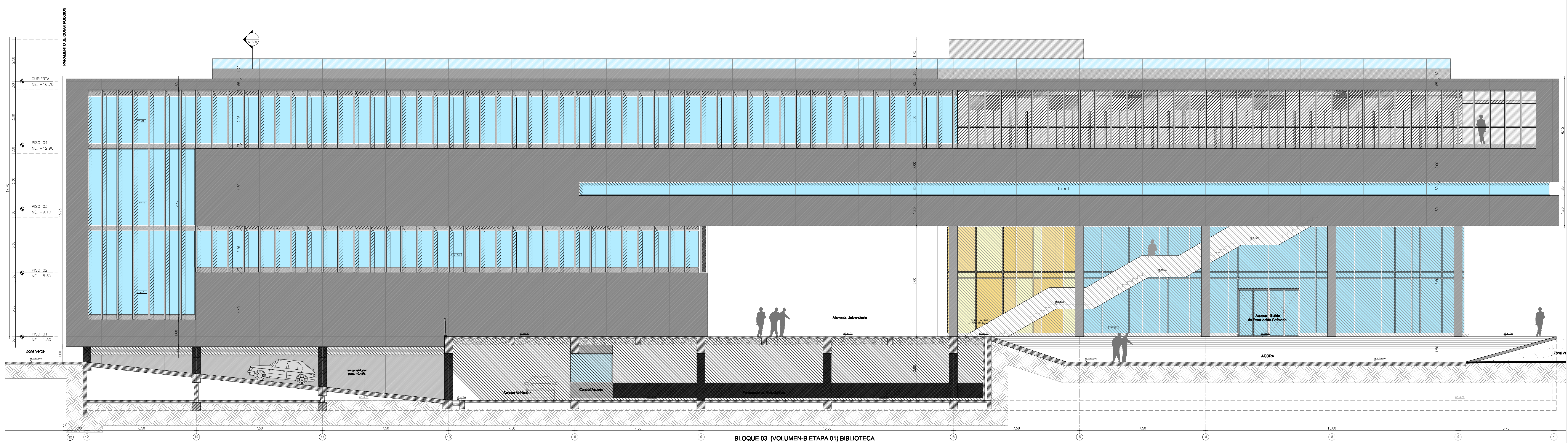
1 FACHADA 01 - NorOcc FRENTE A BLOQUE A ESCALA: 1:100 BLOQUE 03 (VOLUMEN-B ETAPA 01) Ed. de AUDITORIOS y BIBLIOTECA
