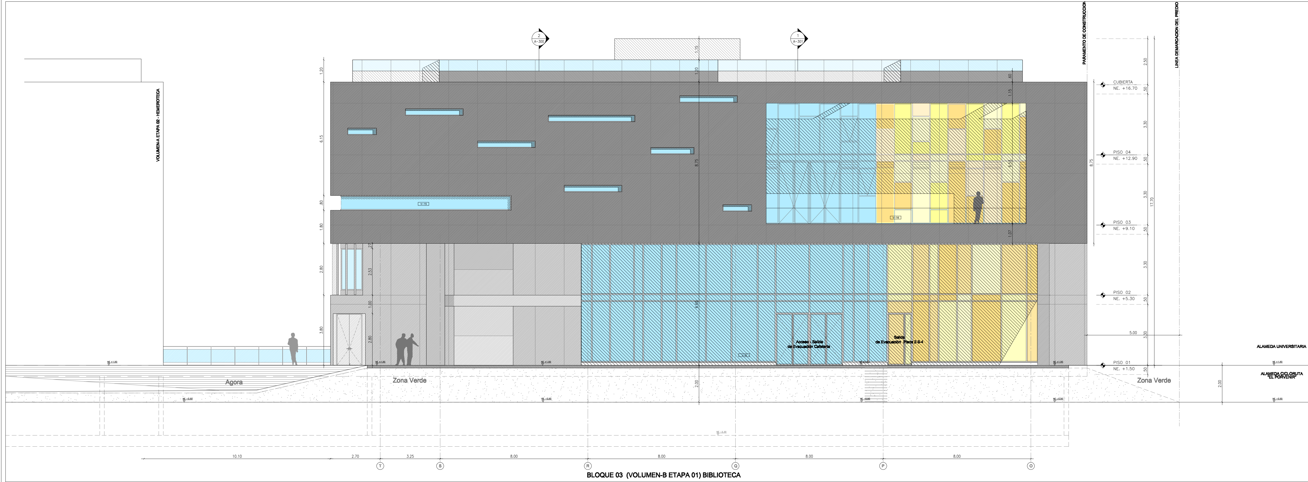
2 FACHADA 02 - SurOcc FRENTE A PARQUE IDR ESCALA: 1:100 BLOQUE 03 (VOLUMEN-B ETAPA 01) Ed. de AUDITORIOS y BIBLIOTECA
