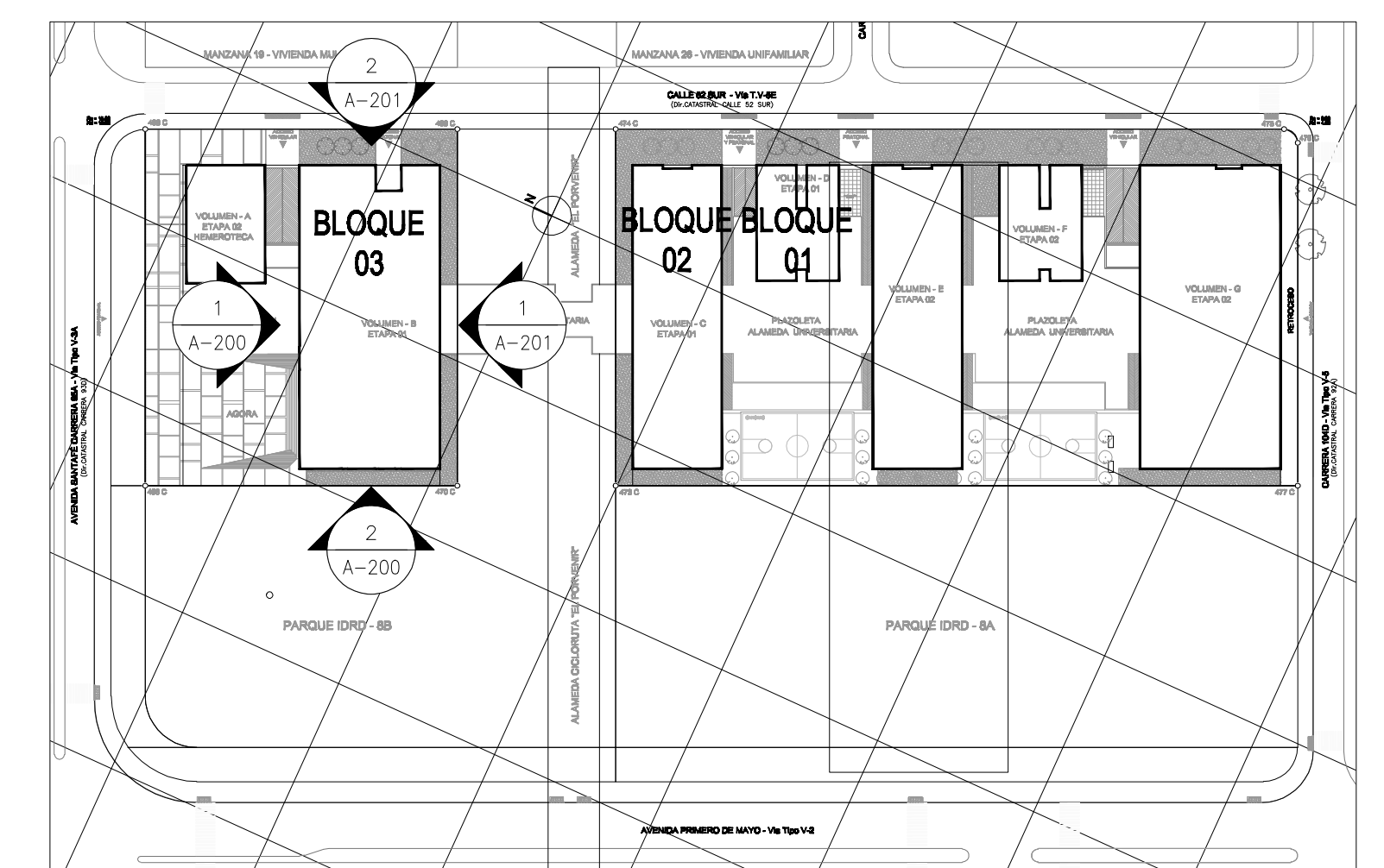
3 LOCALIZACION FACHADAS
