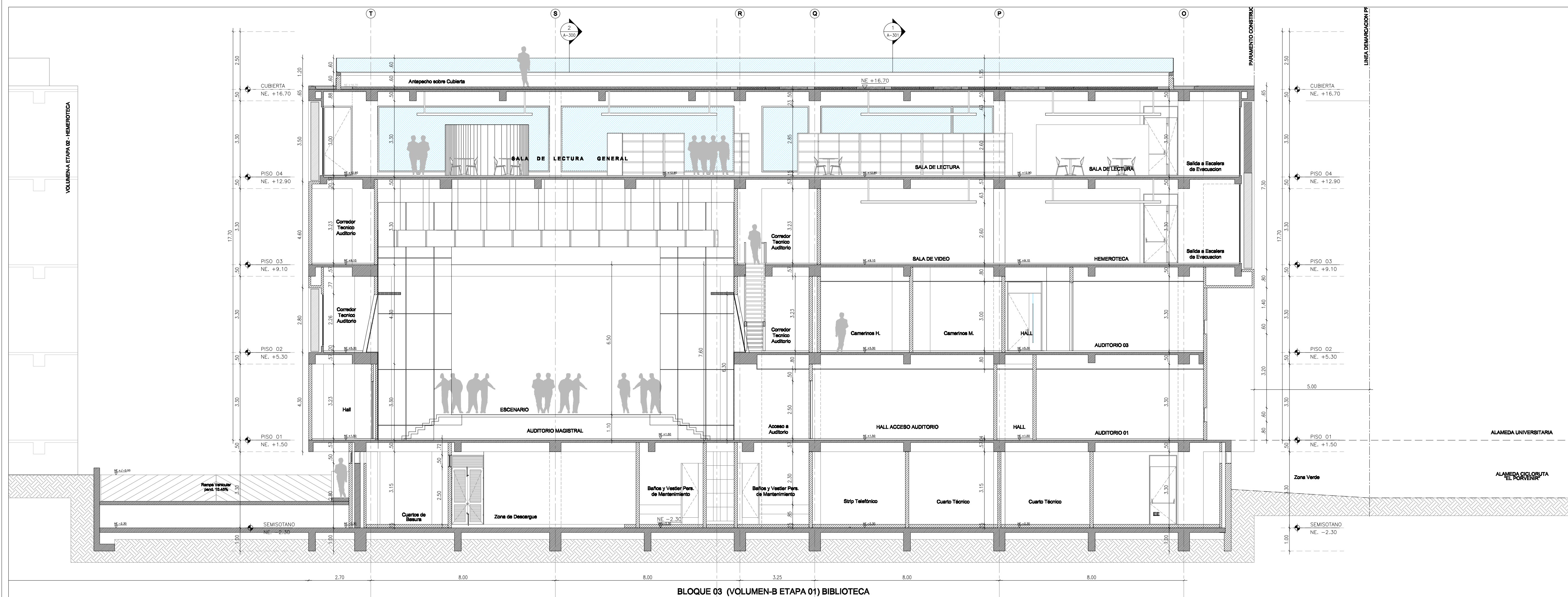
1 CORTE A-A' TRANSVERSAL ESCALA: 1:100 BLOQUE 03 (VOLUMEN-B ETAPA 01) Ed. de AUDITORIOS y BIBLIOTECA
