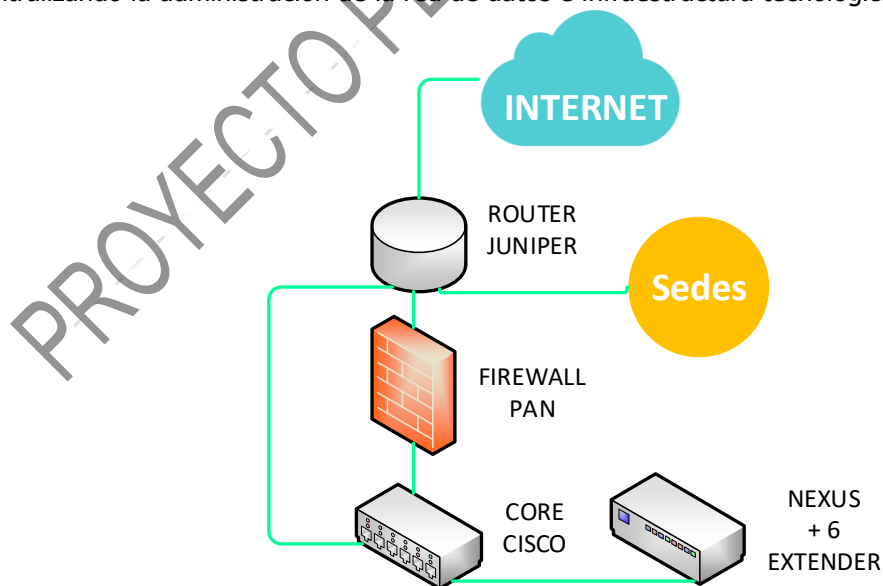
Figura 1: Equipos principales en nodo central. Fuente Red de Datos UDNET
