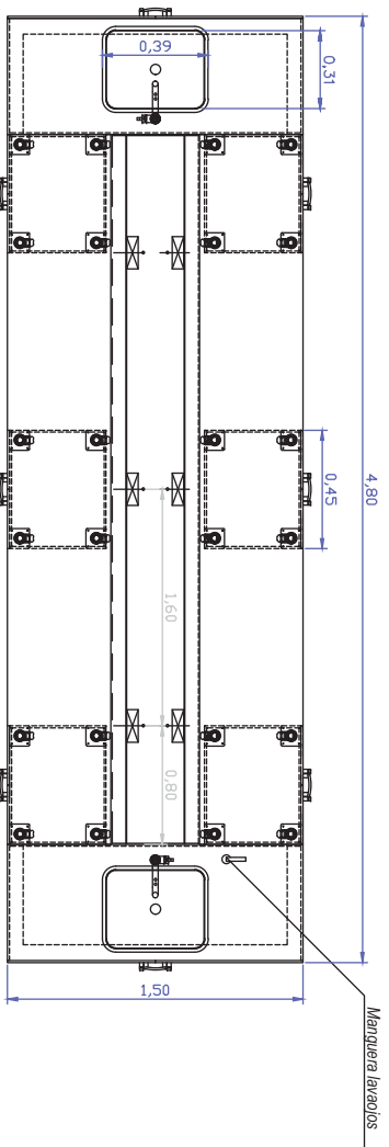
Planta
