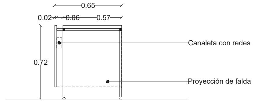
ALZADO LATERAL
