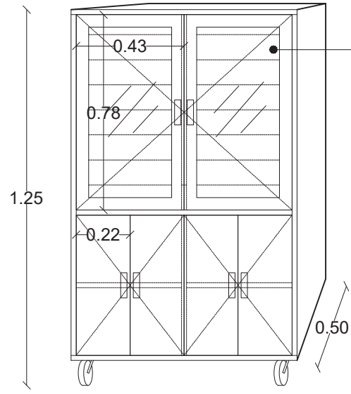
Mueble Cerrado
