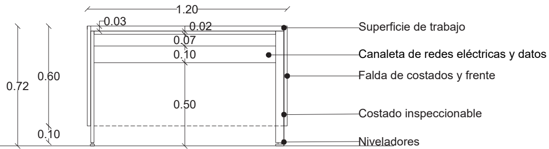
ALZADO FRONTAL
