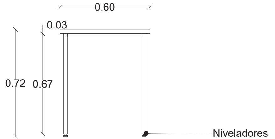
ALZADO LATERAL
