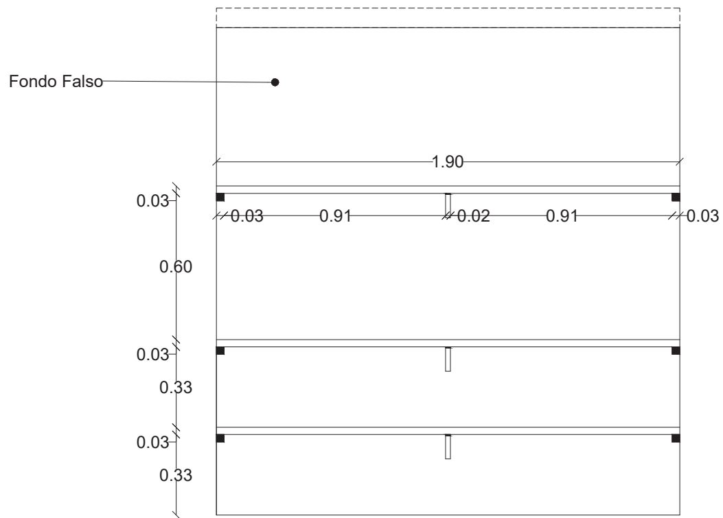
ALZADO FRONTAL
