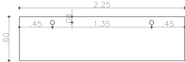
VISTA EN PLANTA SUPERFICIE
