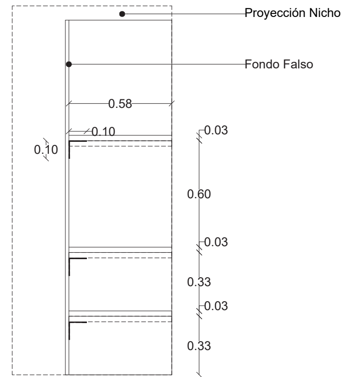
ALZADO LATERAL
