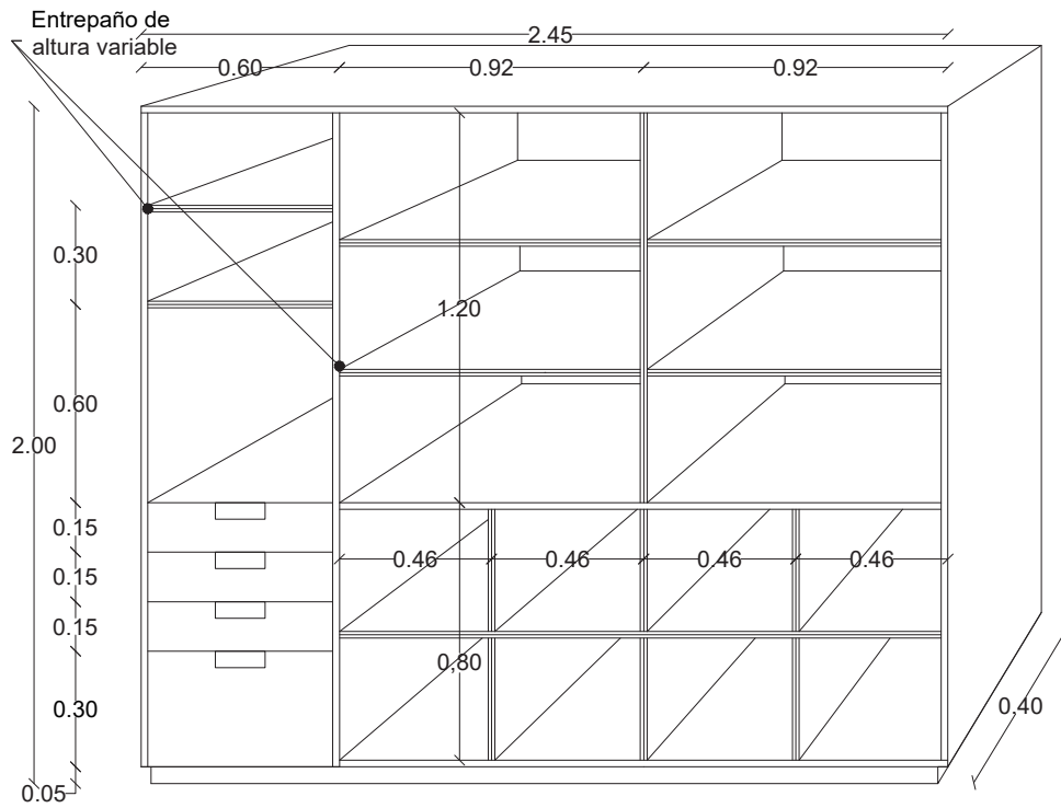
Mueble abierto
