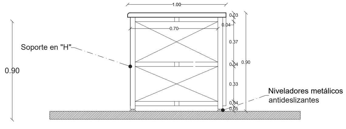
Mueble interior
