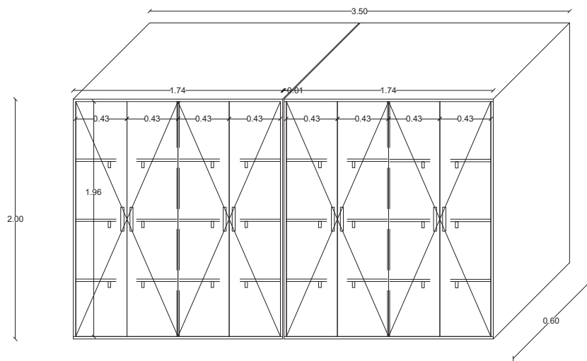
Mueble Cerrado
