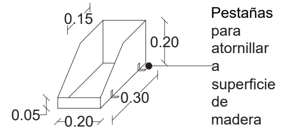
Detalle soporte de Tamiz
