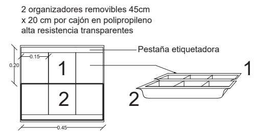
Detalle organizadores cajones grandes
