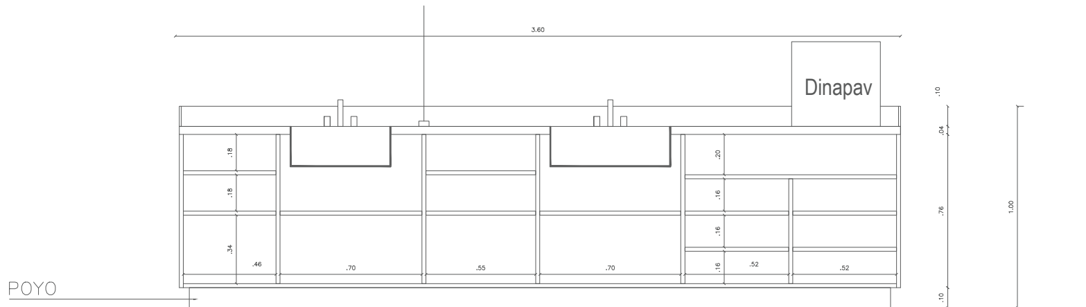
VISTA ALZADO MUEBLE ABIERTO
