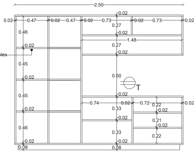
MUEBLE ABIERTO
