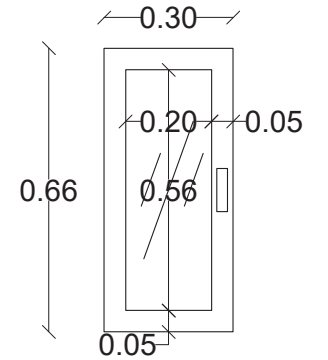
Detalle Puerta
