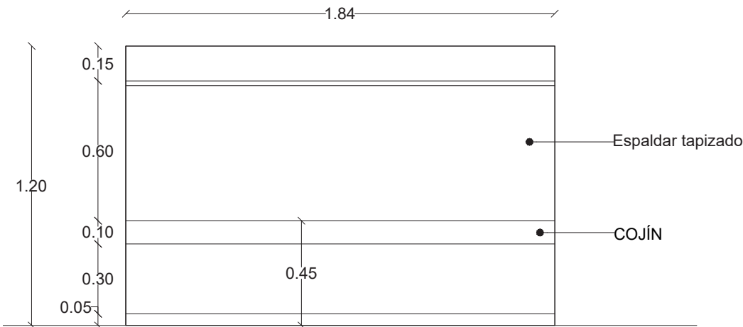
ALZADO FRONTAL
