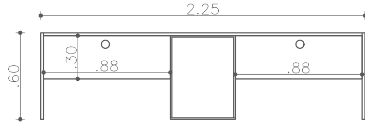
VISTA EN PLANTA BAJO SUPERFICIE
