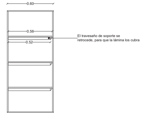
Vista Lateral
