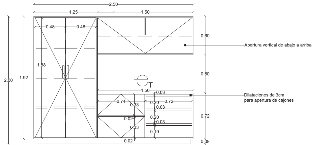
MUEBLE CERRADO
