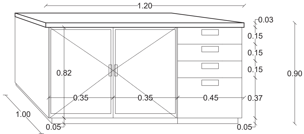
Mueble Exterior
