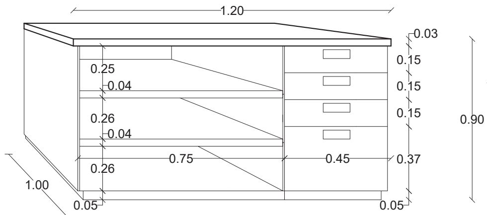
Mueble interior
