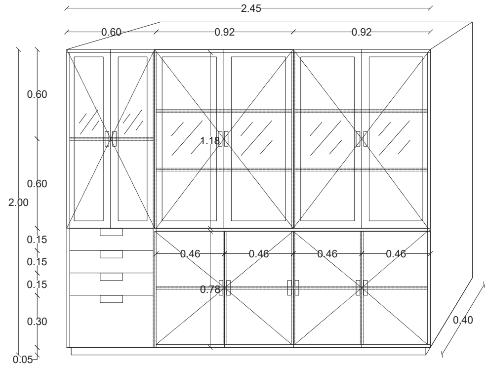
Mueble Cerrado
