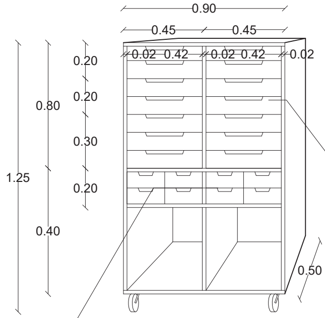
Mueble abierto
