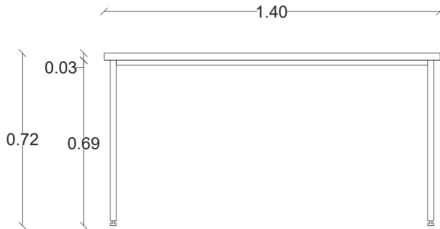
ALZADO FRONTAL
