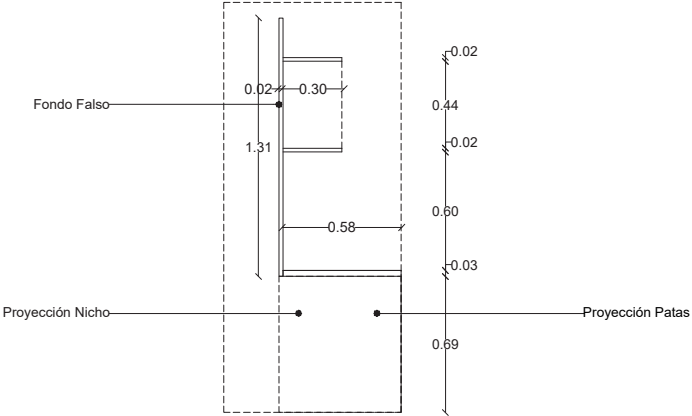
ALZADO LATERAL
