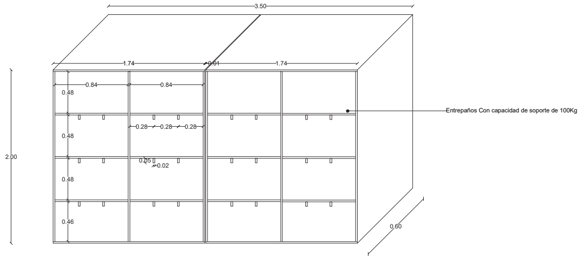
Mueble Abierto
