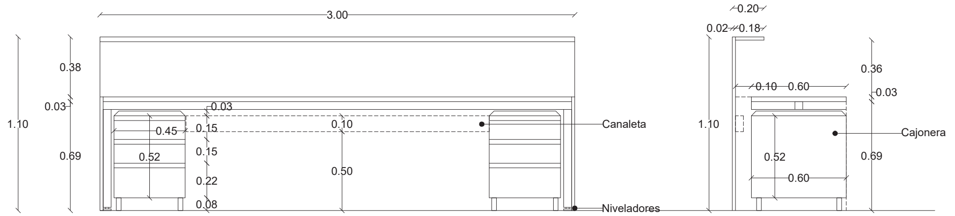
Alzado Frontal
