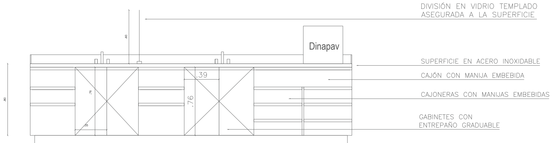
VISTA ALZADO MUEBLE CERRADO
