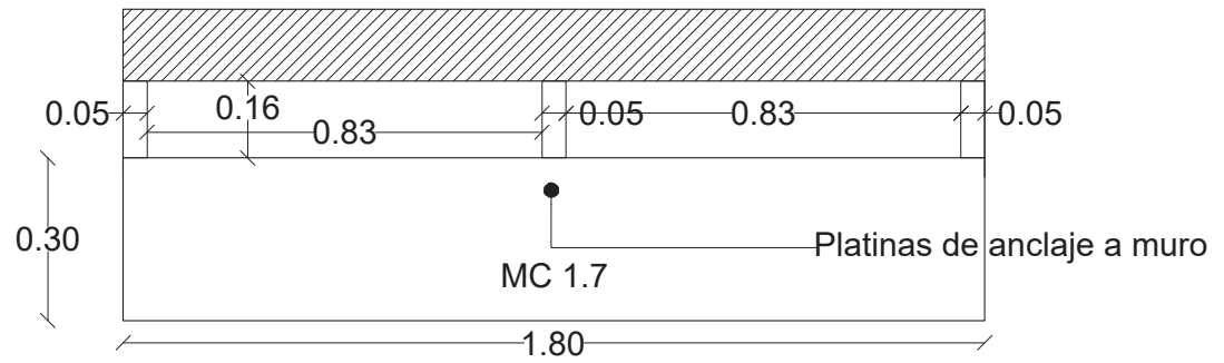
Detalle Puerta
