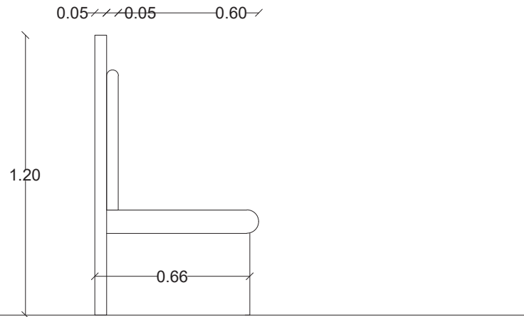
ALZADO LATERAL
