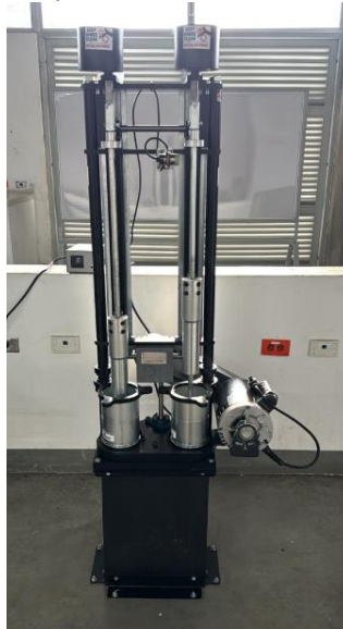
Ilustración 1. Compactador Marshall de doble martillo.
